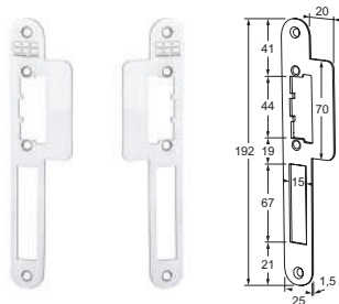
50LPL lange afgeronde lipsluitplaat DIN links 50LPR lange afgeronde lipsluitplaat DIN rechts
